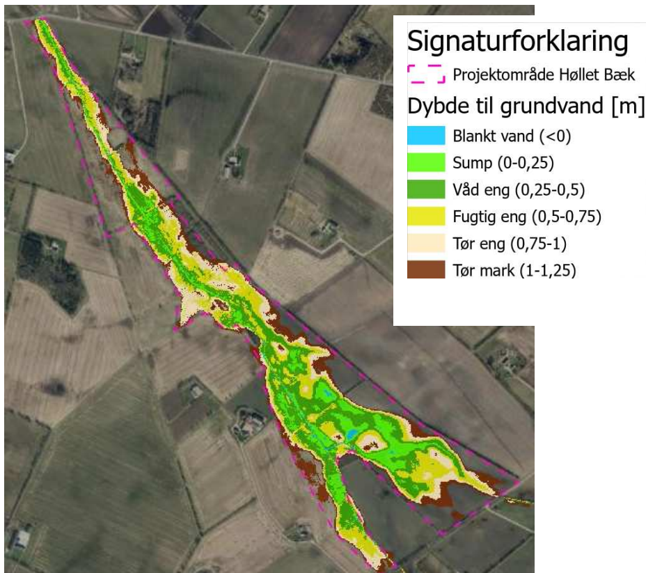
Fig. 2 Afvandingsforhold ved projektrealisering
