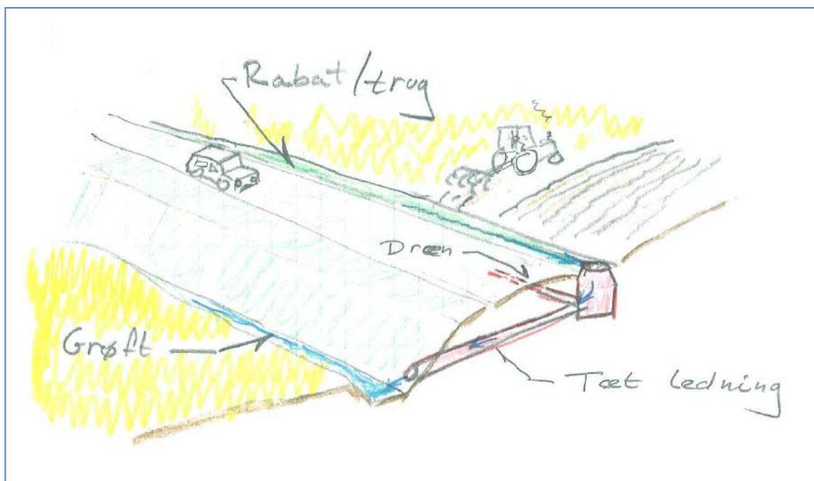
Principskitse for vejafvanding i landområde
